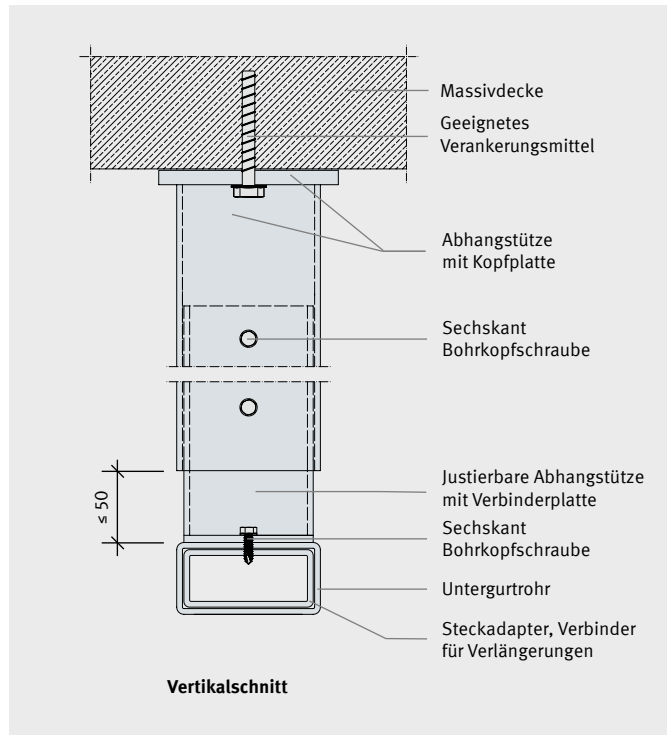
Anschluss an Massivdecke; Abhangstütze mit justierbarem Unterteil
