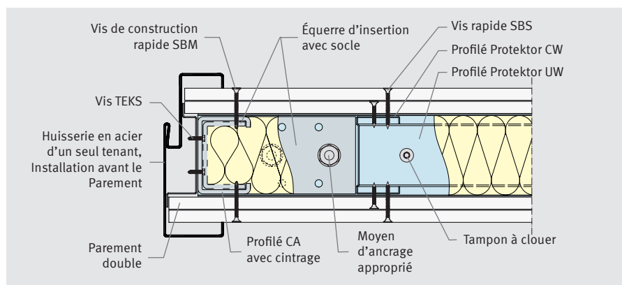
Plan d'ensemble – montage d'une huisserie en acier d'un seul tenant, vissage simple et rapide dans le profilé CA
